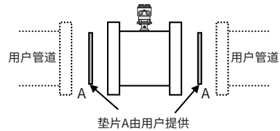
图3.3.2 无接地环的安装
