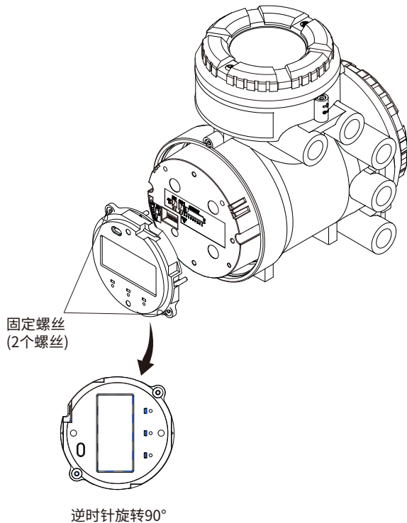
图3.6.2 将显示单元方向改变90°
