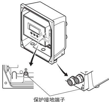
图4.4.6 保护接地端子的位置(AXFA11分体型变送器)
