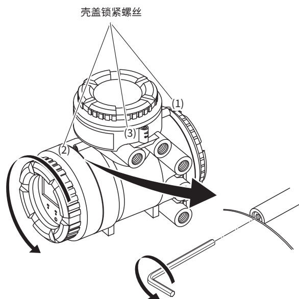
图4.4.7 取下AXW4A分体型变送器的接线盒盖
