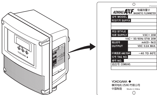
图2.4 铭牌(AXFA11分体型变送器)
