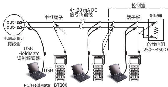
图5.6 连接BRAIN配置工具
