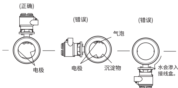
图3.1.6 安装方向
