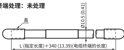
图4.2.3 信号电缆的电缆终端
