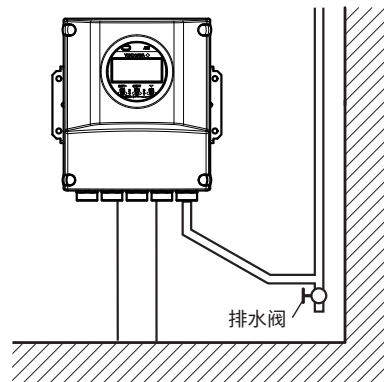
图4.3.3 分体型变送器(AXG1A/AXFA11)
