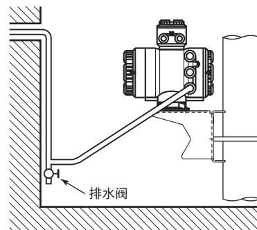
图4.3.2 分体型变送器(AXW4A)
