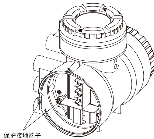
图4.4.4 保护接地端子的位置(AWX4A分体型变送器)
