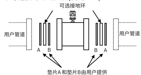
图3.3.3 带接地环GR1的安装
