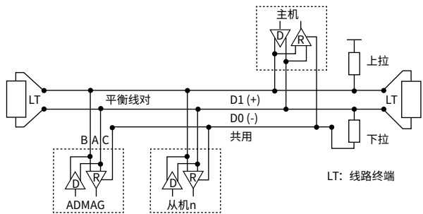
图6.3.2 Modbus连接
