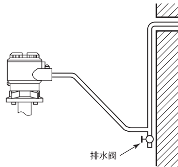
图4.3.1 分体型传感器
