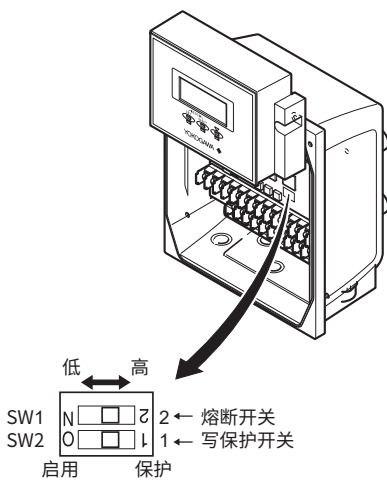
图6.3.6 硬件开关
