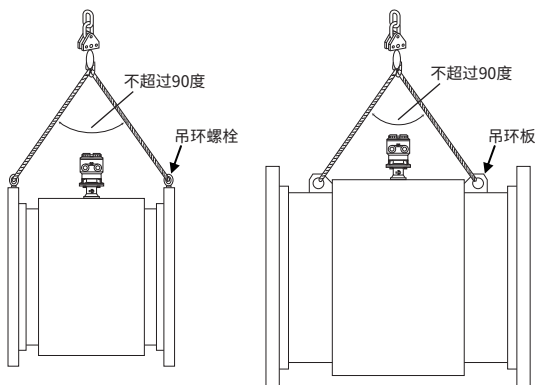
图3.2.1 吊起流量计
