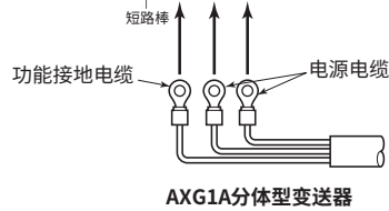
图4.4.1 电源电缆接线
