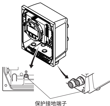
图4.4.5 保护接地端子的位置(AXG1A分体型变送器)
