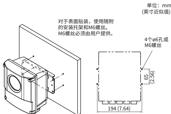
图3.4.3 表面贴装
