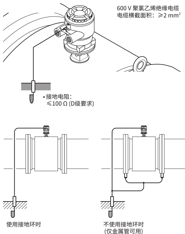
图4.5.6 接地(分体型传感器)
