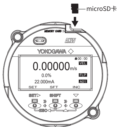
图5.5 microSD设置
